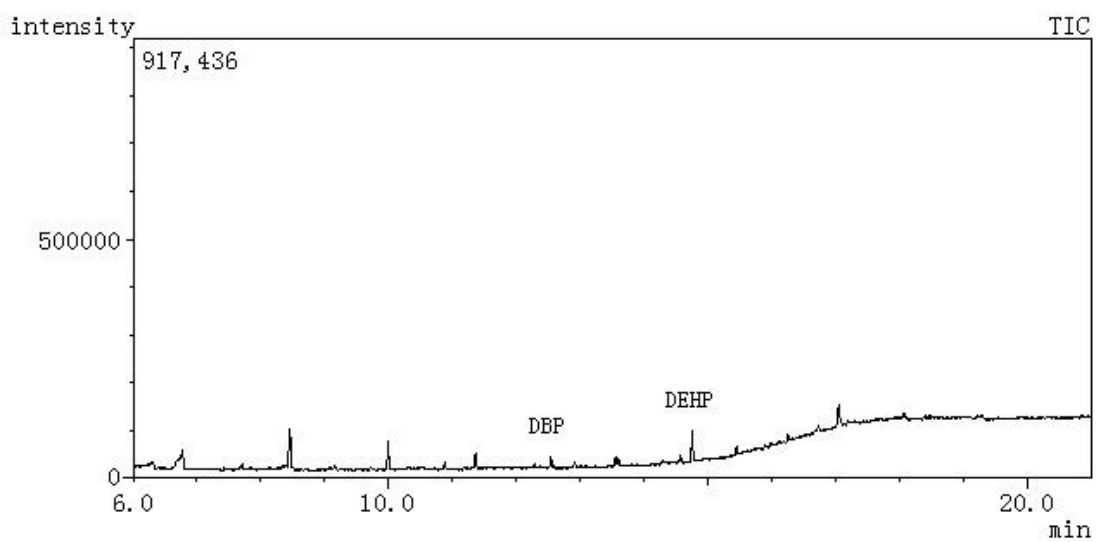
图 5 仪器空白全扫描色谱图 (BDP、DEHP 干扰)
