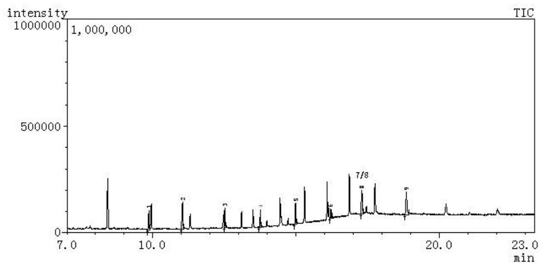
图 9 沉积物样品提取液净化前色谱图
