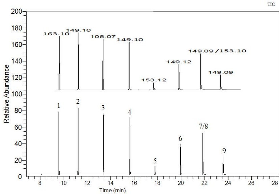
1.邻苯二甲酸二甲酯 (DMP) 2. 邻苯二甲酸二乙酯 (DEP) 3. 苯甲酸苄酯(BBZ) 4.邻苯二甲酸二正丁酯 (DBP) 5. 邻苯二甲酸二戊酯- d_4 (DPP- d_4 ) 6. 邻苯二甲酸二丁基苄酯 (BBP) 7.邻苯二甲酸二(2-乙基己基)酯- d_4 (DEHP- d_4 ) 8. 邻苯二甲酸二(2-乙基己基)酯 (DEHP) 9. 邻苯二甲酸二正辛酯 (DOP)
