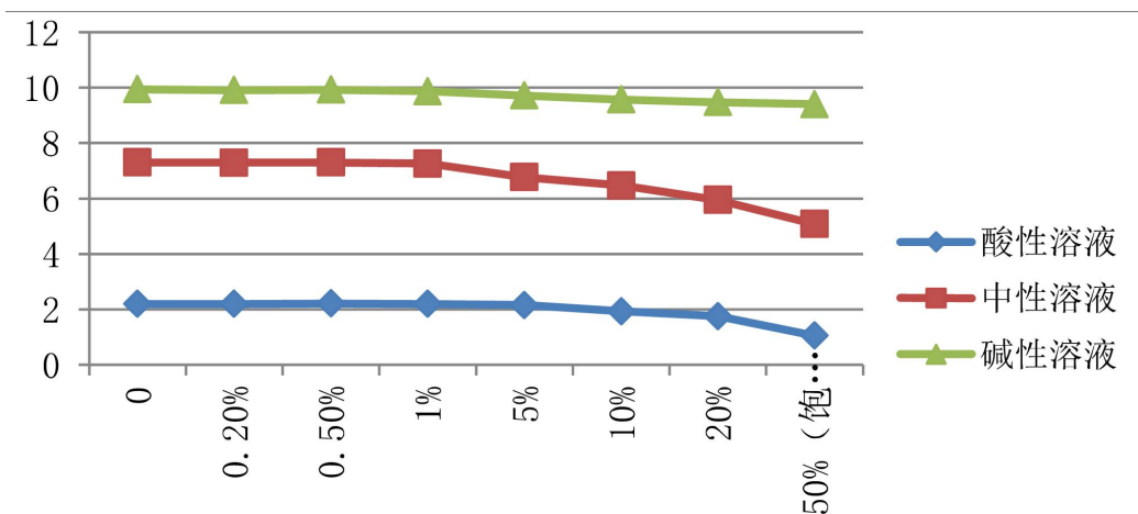
图9 耐高盐电极测定结果
