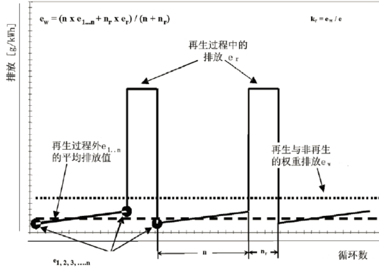
图B.4 再生过程测试示意图
