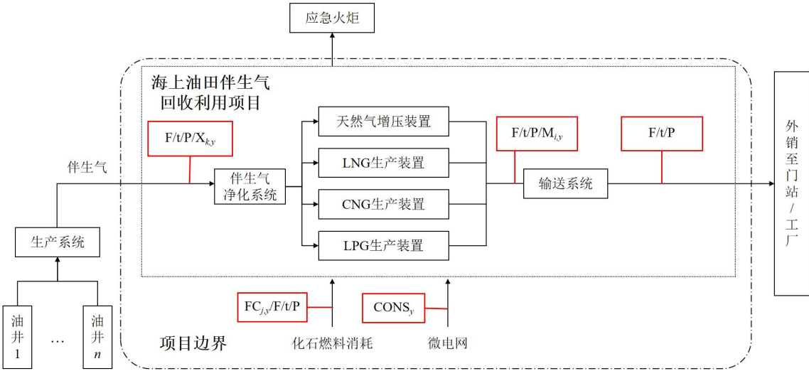
图 2 项目监测点布置示意图
