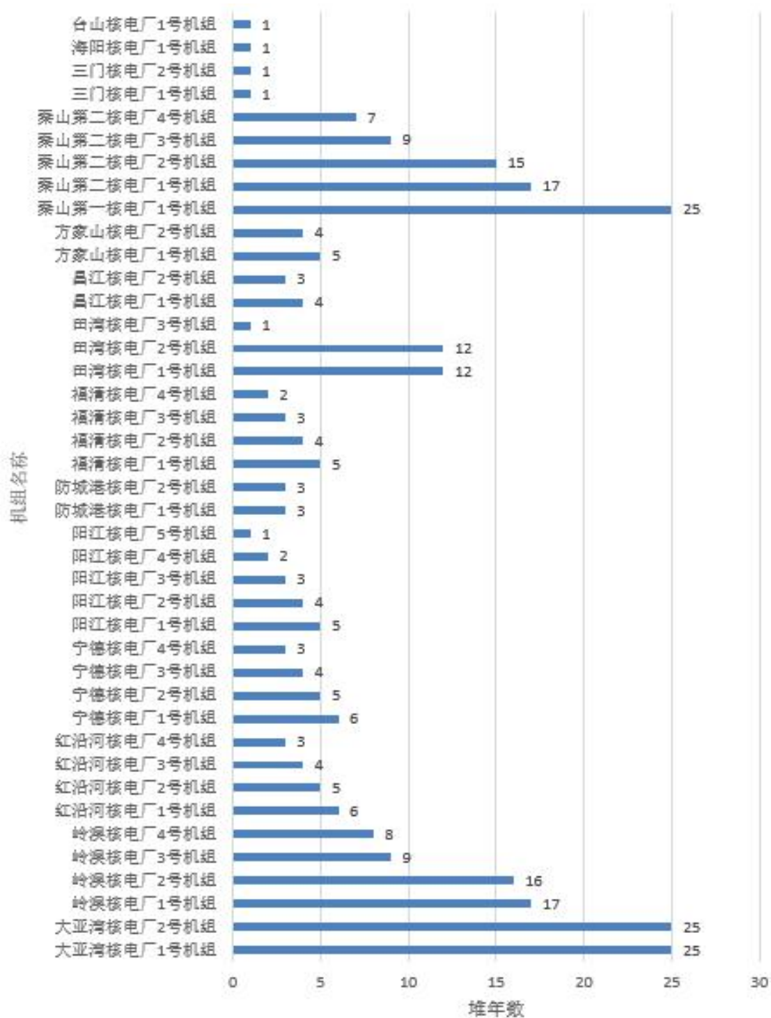
图1 各核电机组堆年数统计（截至2018年底）
