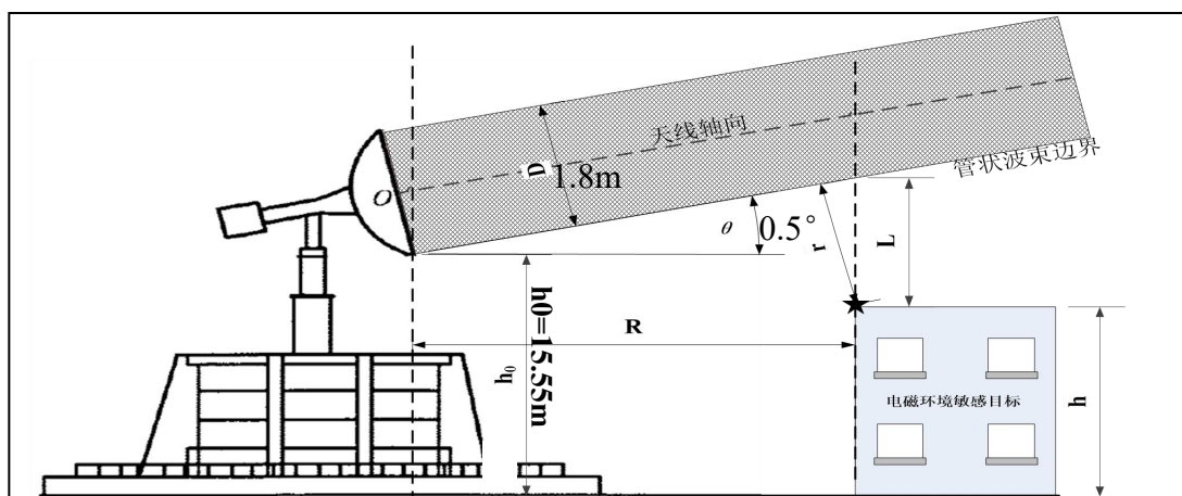
图 4-1 偏轴方向功率密度计算示意图
