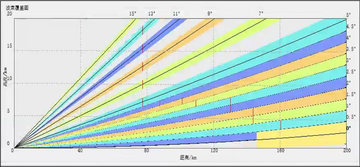
图 2-3 项目雷达设备波束覆盖图
