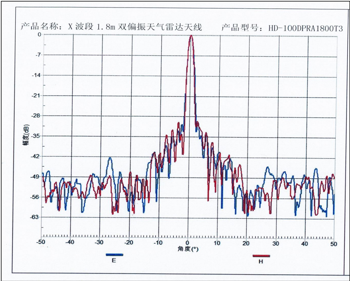
图 2-4 9.4GHz 频率下的天线方向图
