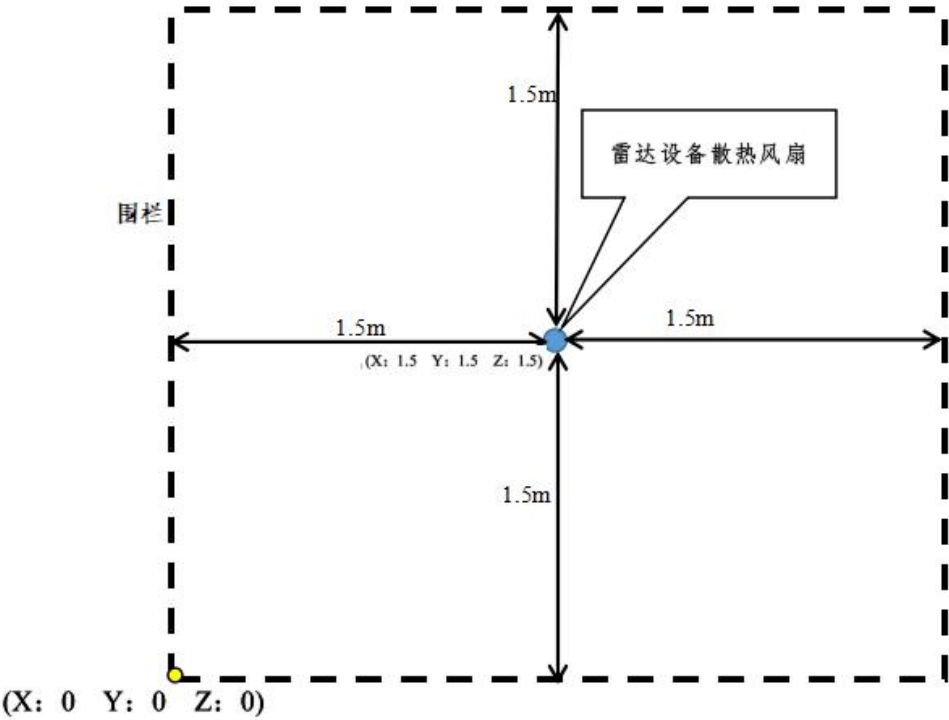
图 4-1 项目单个雷达站噪声主要设备空间位置示意图
