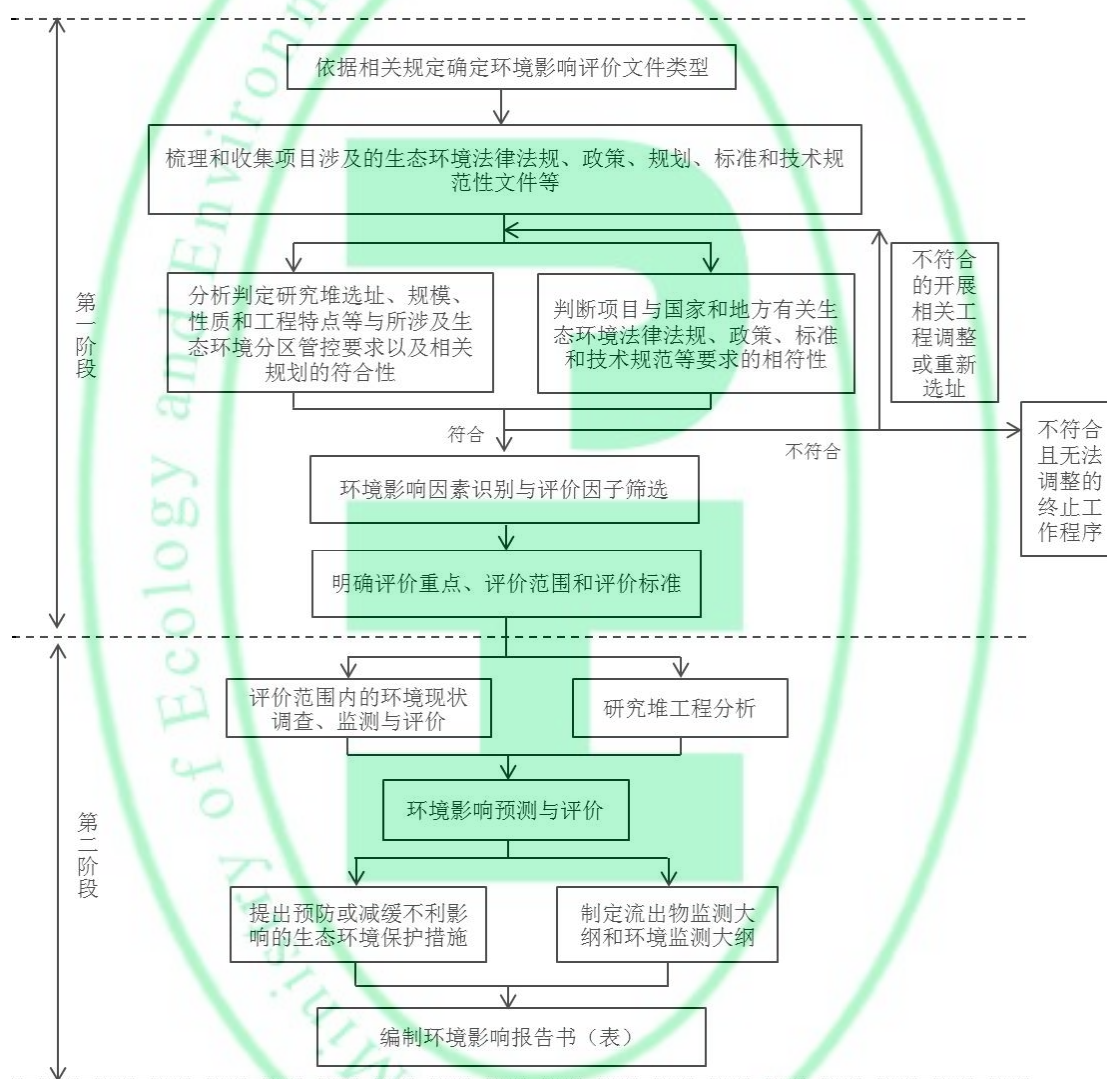
图 1 研究堆环境影响评价工作程序图
