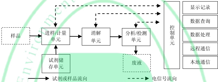
图 1 水质总磷自动监测仪的基本组成单元示意图
